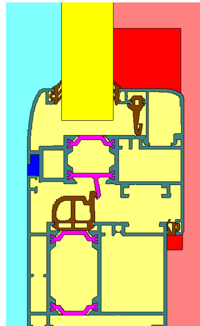
Bild 2 Simulationsmodell
